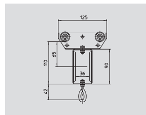
Vodící vozík. Objednací č.: 023295
