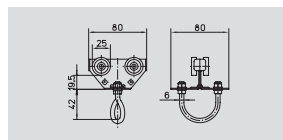
Vozík. Objednací č.: 023293 Kolečko: Kuličkové ložisko pozinkované Nosnost: 20 kg
