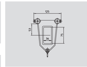
Vodící vozík. Objednací č.: 023905 Provedení: Kolečko i kluzné ložisko z plastické hmoty Nosnost: 6,3 kg
