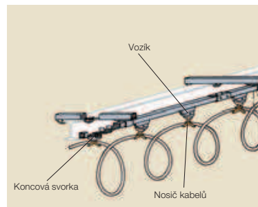
Vodící vozík. Objednací č.: 023295
